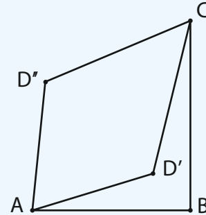
படம் T3 ப-ப-ப-ப-கோ ஊகத்தை நிராகரித்தல்
