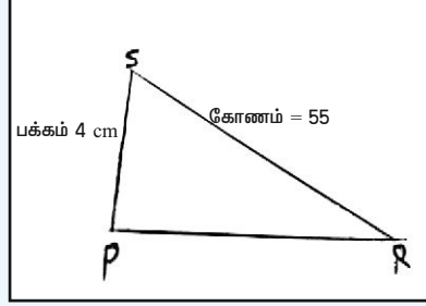
படம் T1 ஒரு முக்கோணத்தை குறிக்க மாணவர்கள் பயன்படுத்தும் வழிமுறை
