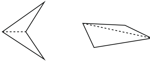
படம் 1 நாற்கரங்களை முக்கோணமாக்கல்
